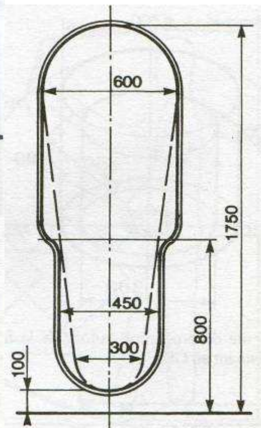
Fig. 4-12. - Côtes d'une ouverture (passage porte) oblique.
