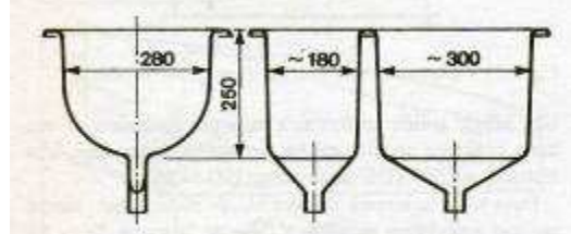
Fig. 7-13 • Vue en coupe transversale et longitudinale d'un évier double réellement adapté à la navigation en mer à la voile.
