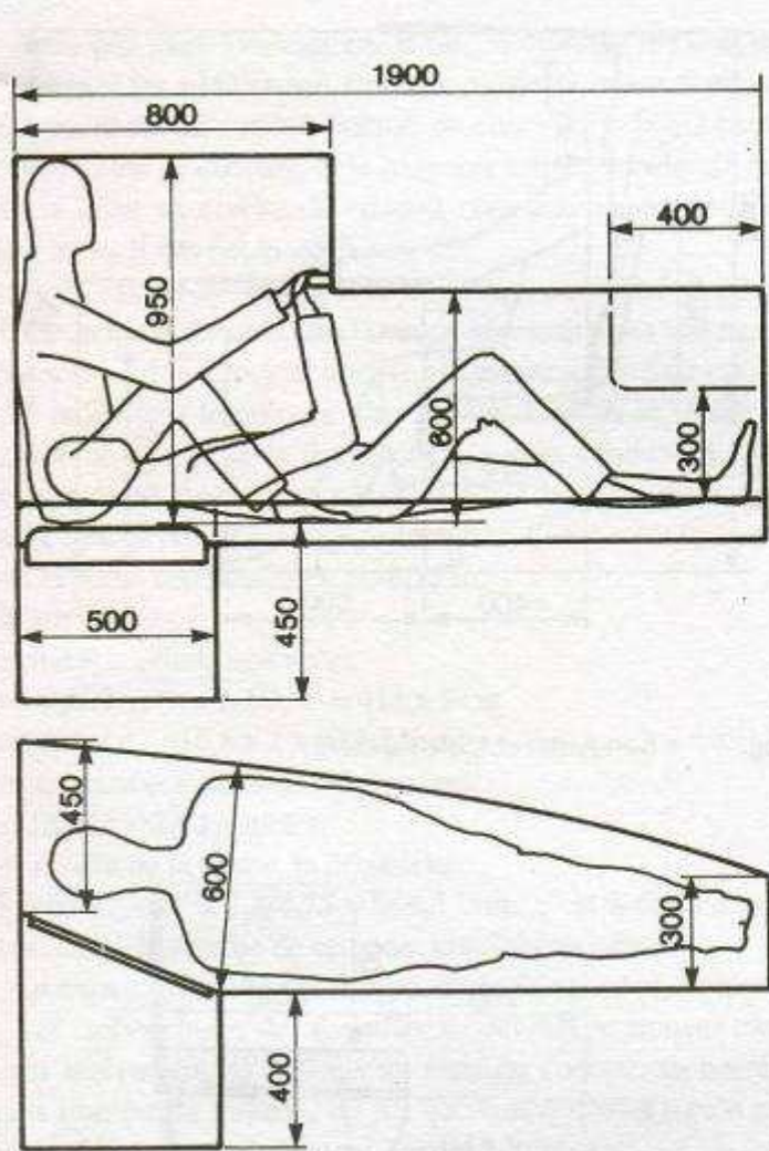
Fig. 7-9 • Dimensions d'une couchette de quart.
