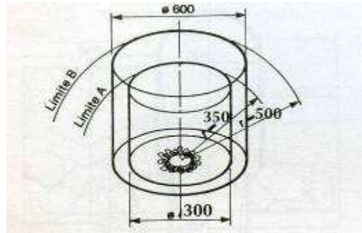
Fig. 7-12 • Limite de protection autour de la flamme d'un réchaud fonctionnant au GPL.
