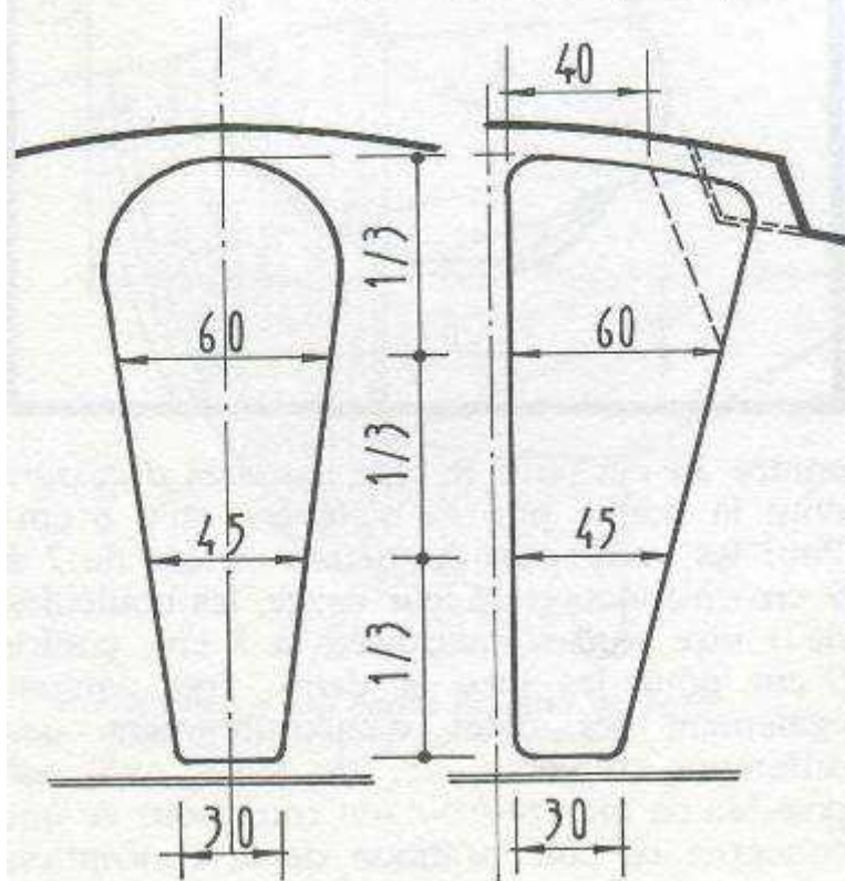
Fig. 4-12. - Côtes d'une ouverture (passage porte) oblique.
