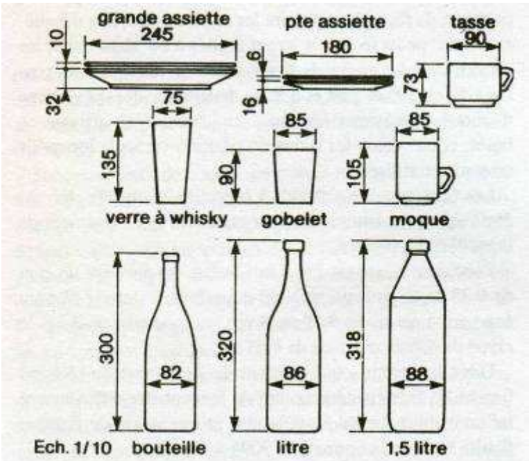
Fig. 7-14 • Dimensions de quelques objets de vaisselle et bouteilles.
