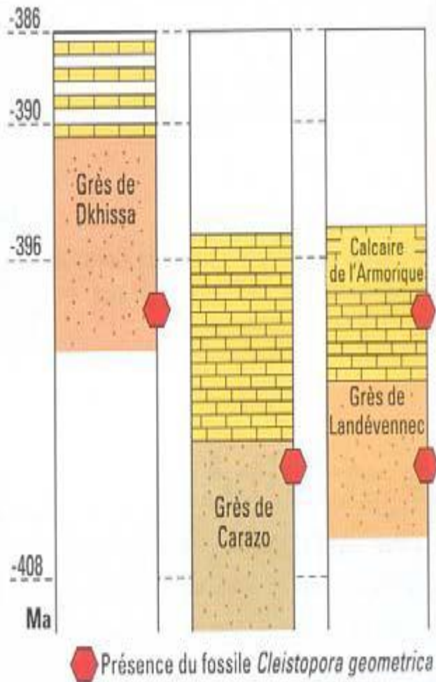
3 Colonnes stratigraphiques montrant la position de Cleistopora geometrica en France, en Espagne et en Algérie.
