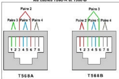
Schéma des codes de couleurs utilisés pour les câbles T568-A et T568-B
