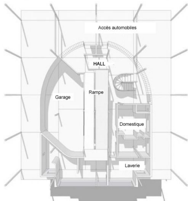
Rez-de chaussée « villa Savoye »
