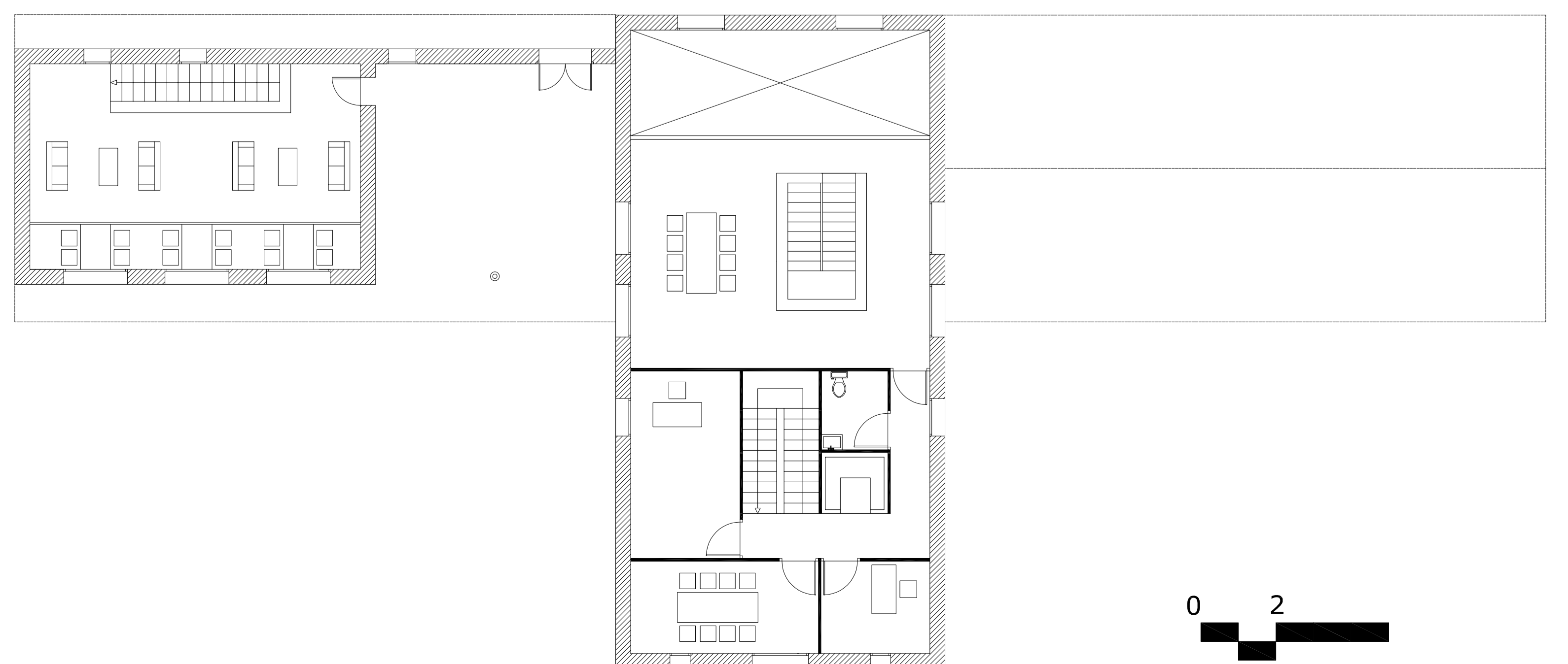
PLAN ETAGE
