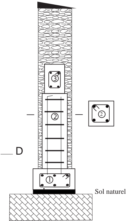
COUPE NORD-SUD EN A-B
