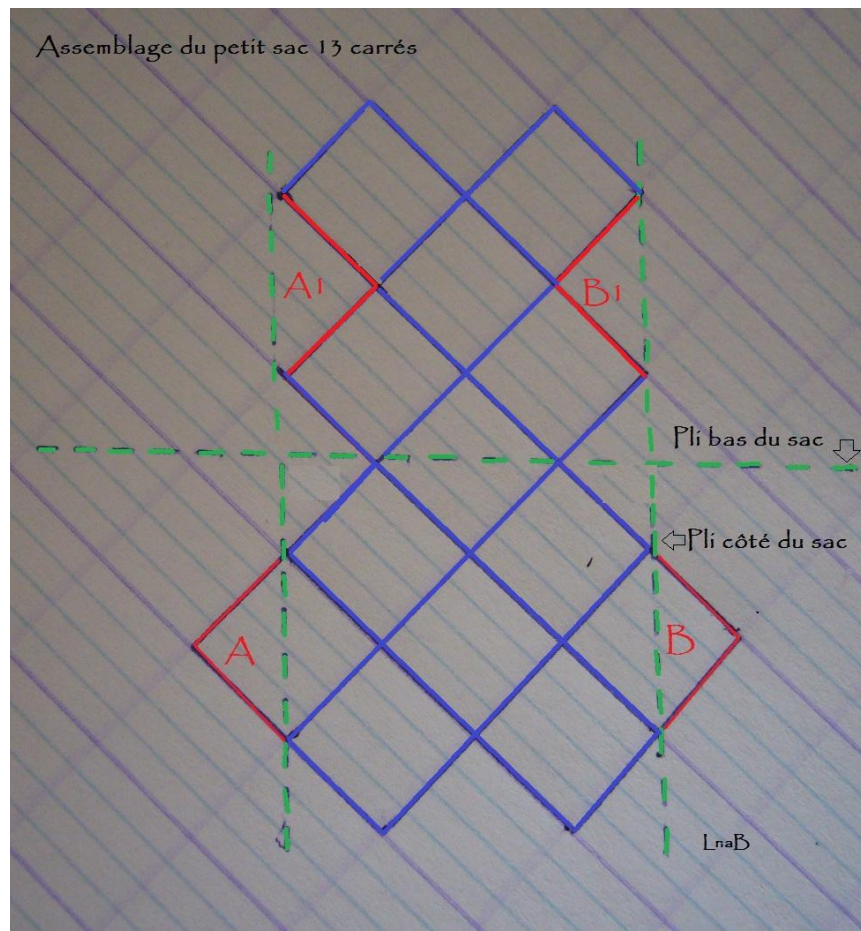
Sac réalisé avec 13 carrés simples
