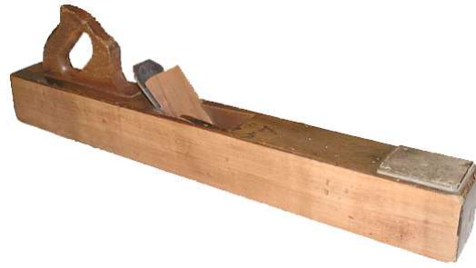
Varlope, rabot à dresser (rendre droit) estampillé : "Garanti Véritable CORMIER" (bois dur pour outillage).
