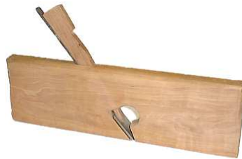
Guillaume, rabot étroit pour rainures. Le fer a la même largeur que le rabot ; le copeau s'évacue sur le côté et non sur le dessus (Longueur = 28 cm ; largeur = 2 cm).
