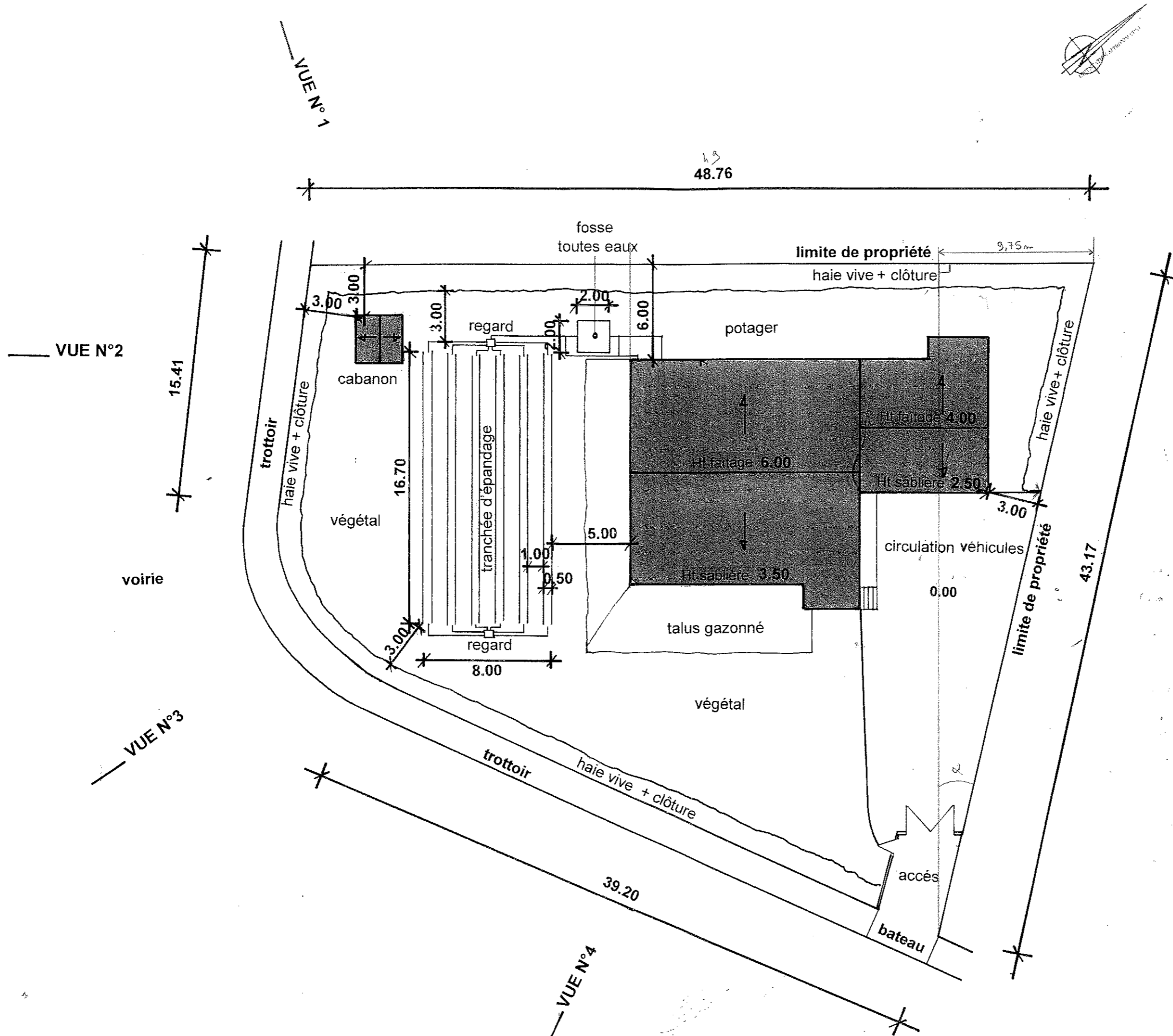
PLAN DE MASSE Echelle 1/250 e
