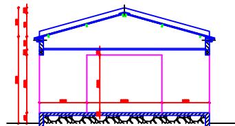
FACADE ARRIERE (OUEST/EST)
