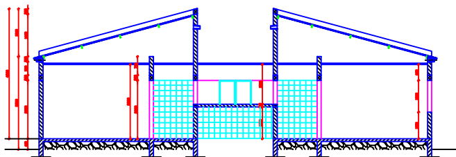
COUPE (FACADE ARRIERE) (OUEST/EST)
