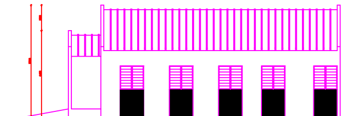
FACADE LATERALE GAUCHE (NORD/SUD)
