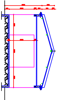
FACADE ARRIERE (OUEST/EST)
