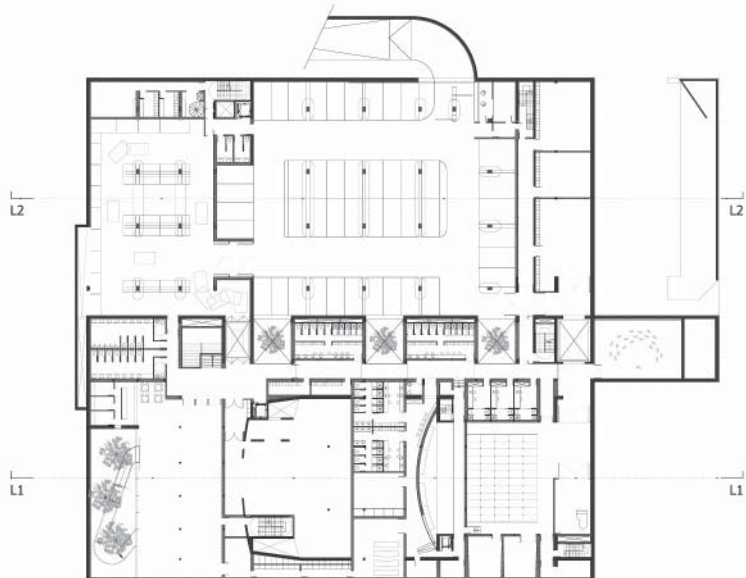
NIVEAU -1 - PARKINGS, ENTREPOTS SCENIQUES ET INSTALLATIONS
