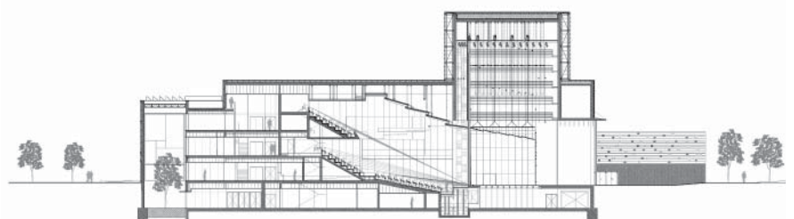
COUPE L1 SUR LE PATIO ET LA SALLE PRINCIPALE
